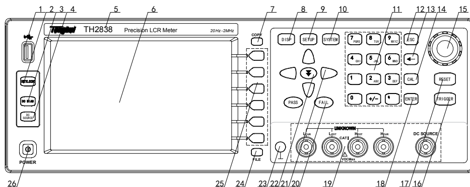
图 2-1. 前面板说明
