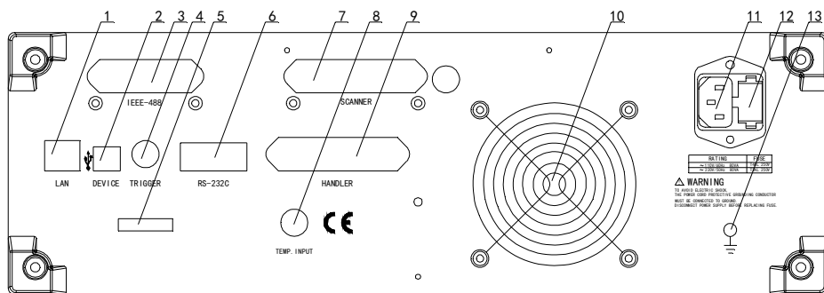
图 2-2. 后面板说明
