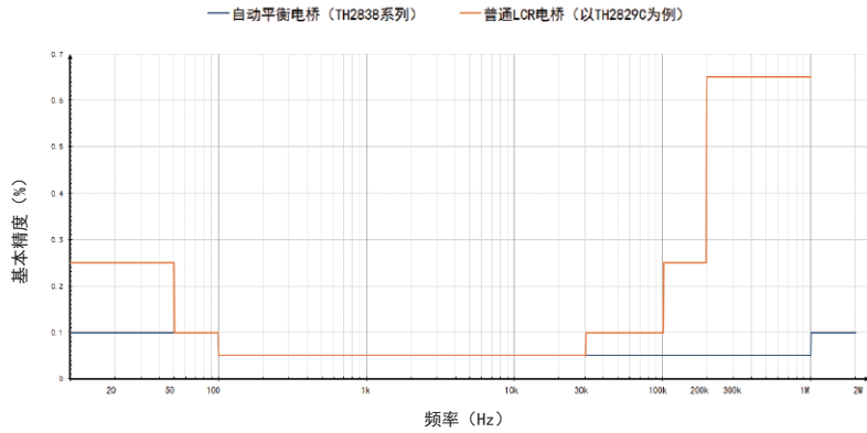
LCR数字电桥精度对比表
